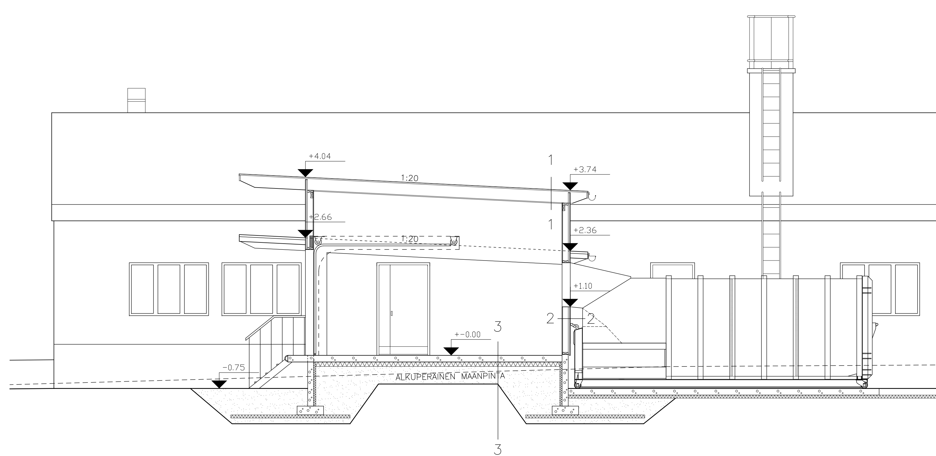
LEIKKAUS A-A
